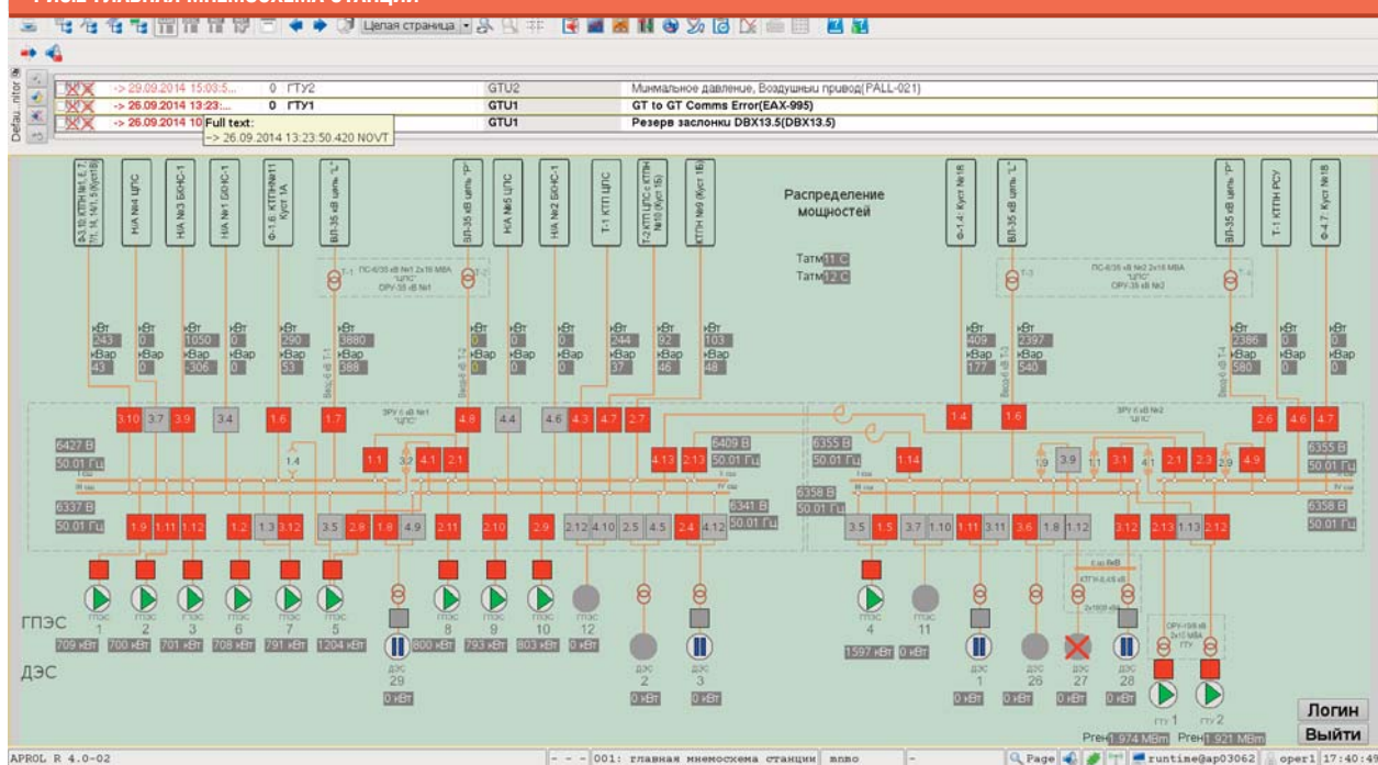
РИС.2 ГЛАВНАЯ МНМОСХЕМА СТАНЦИИ
